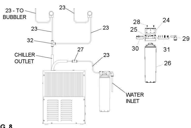
LNTE8C/LNTE8RAC TUBE ROUTING
